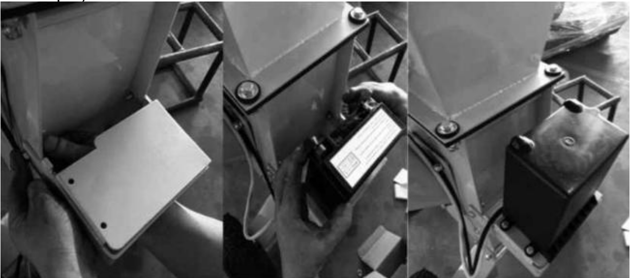
Étape 5 - Choix facultatif (uniquement pour démarreur électrique)
